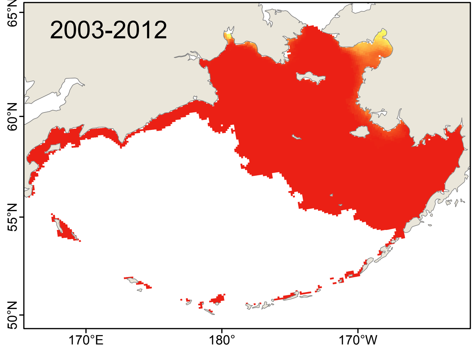
(b) Model: ECHO-G
